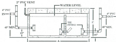
SECTION:ELEVATION
