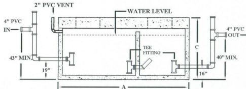
SECTION:ELEVATION
